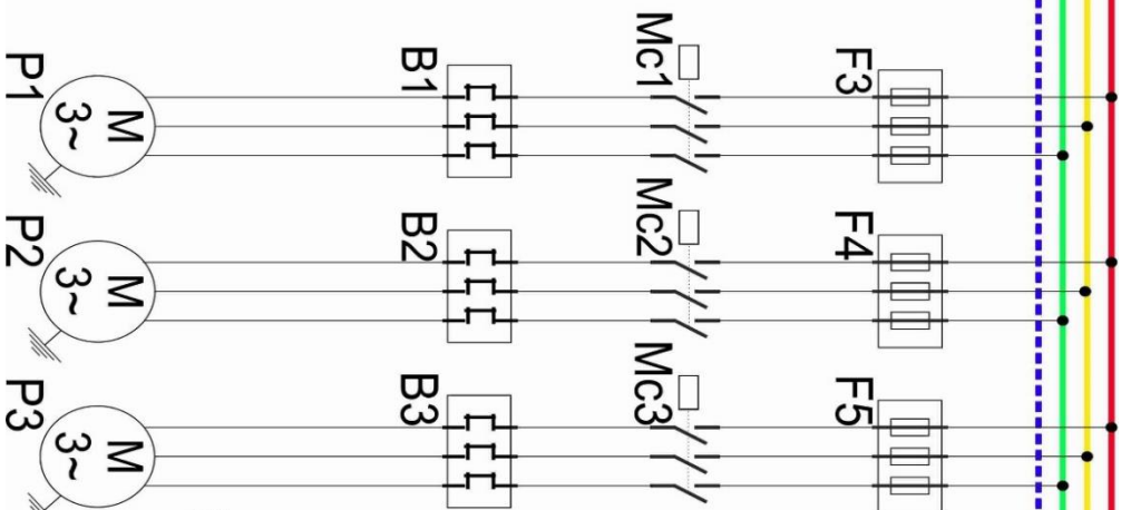
نقشه مدار قدرت در حالت PRESSURE SWITCH
