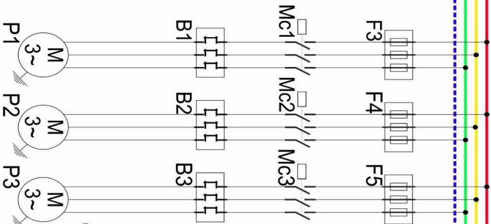
نقشه مدار قدرت در حالت ON/OFF & SENSOR
